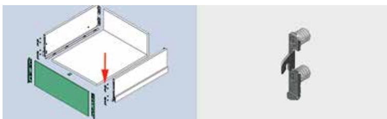
Fixation supérieure pour façades intérieures Scala avec hauteur 186 mm
